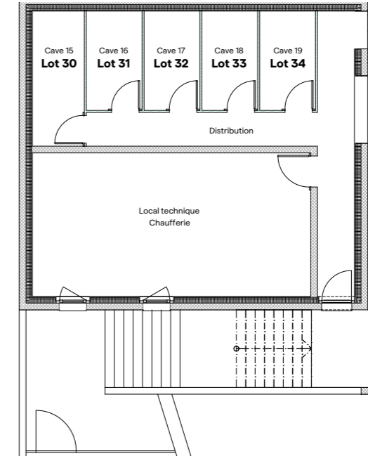
1 er étage
