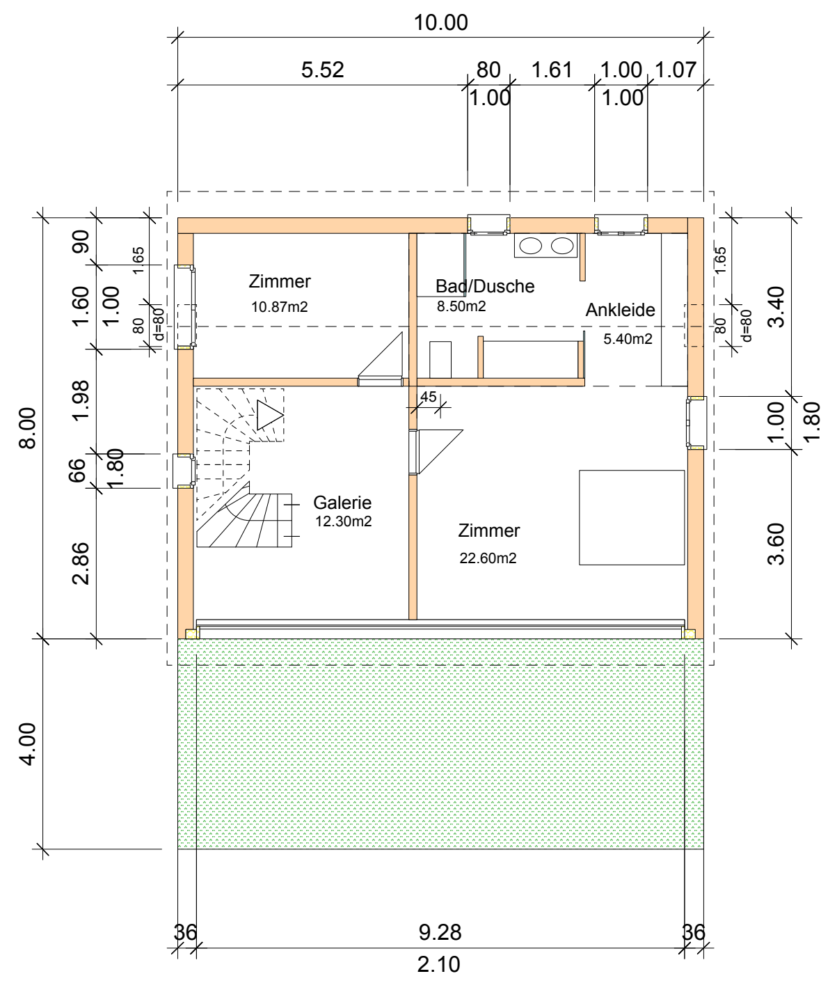
Grundriss Obergeschoss
