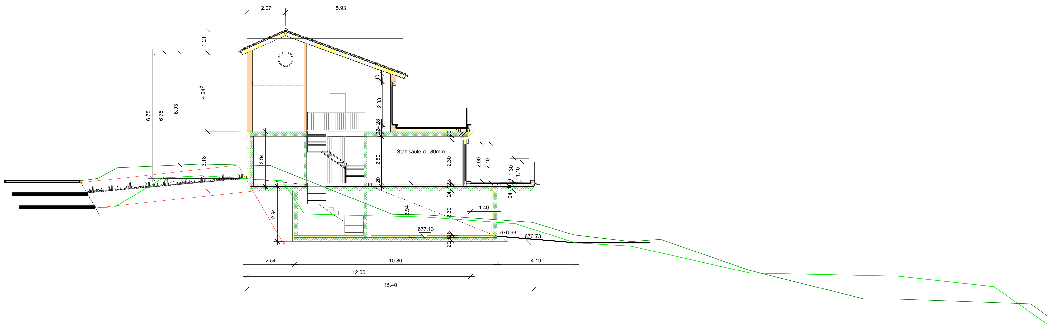
Schnitt A-A
