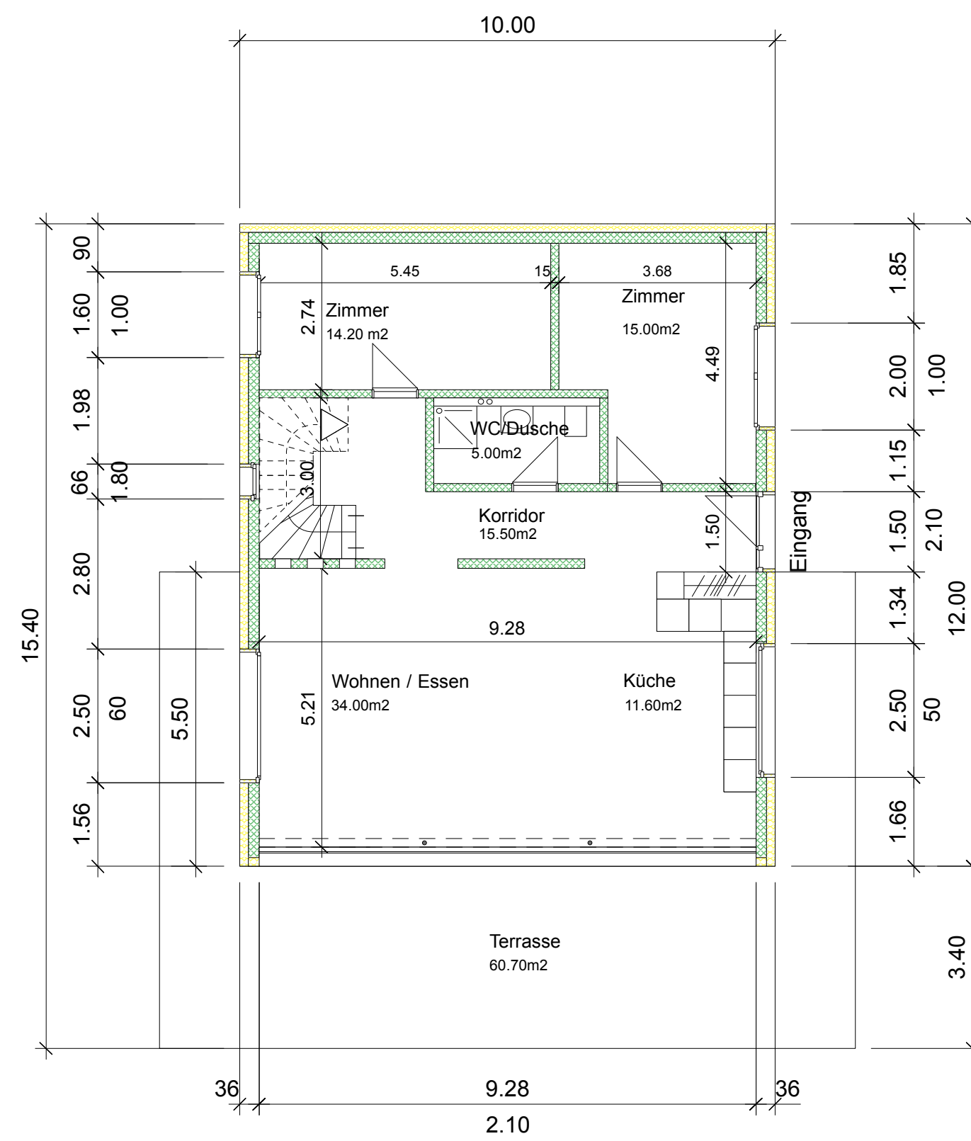
Grundriss Erdgeschoss
