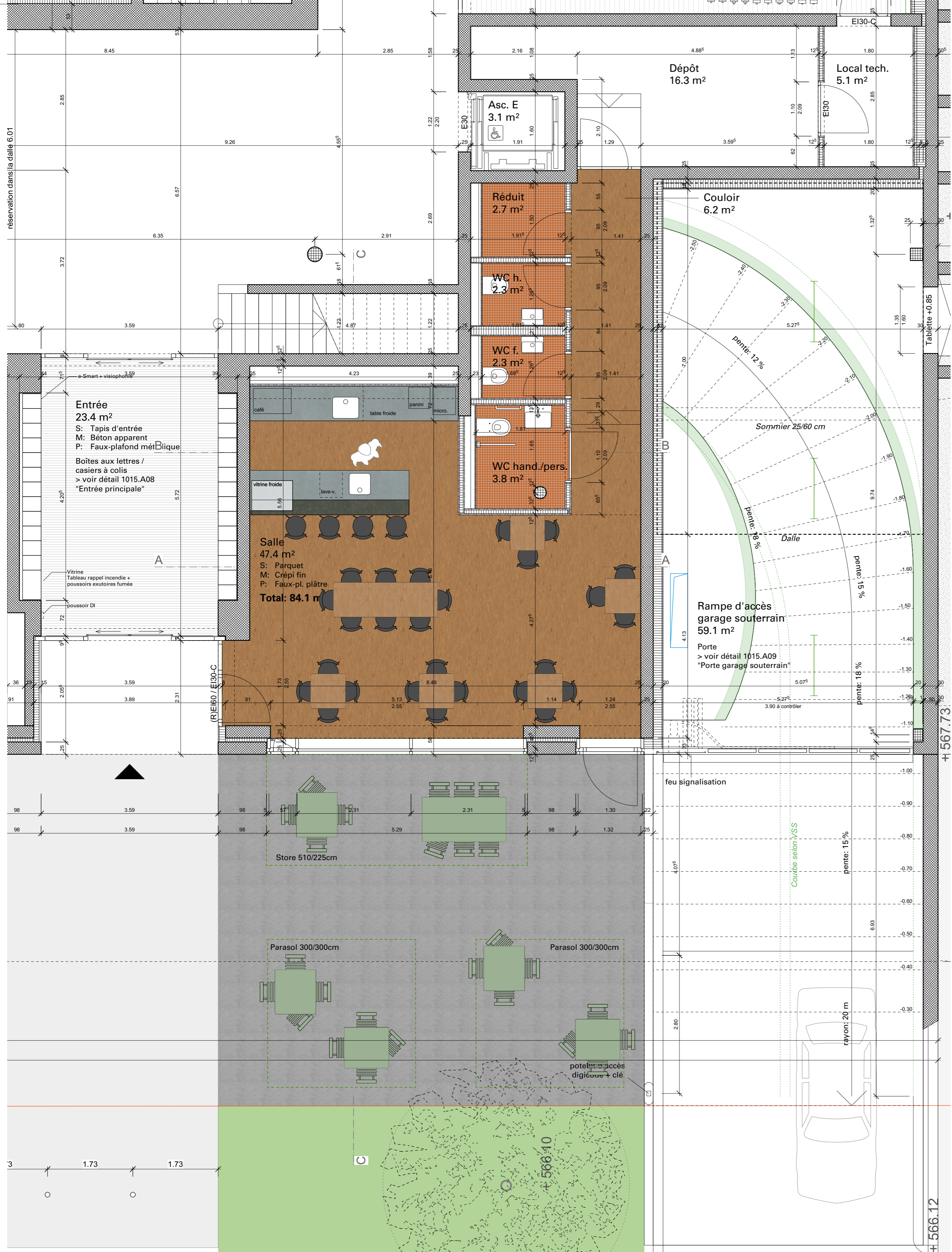
Plan 1:50
