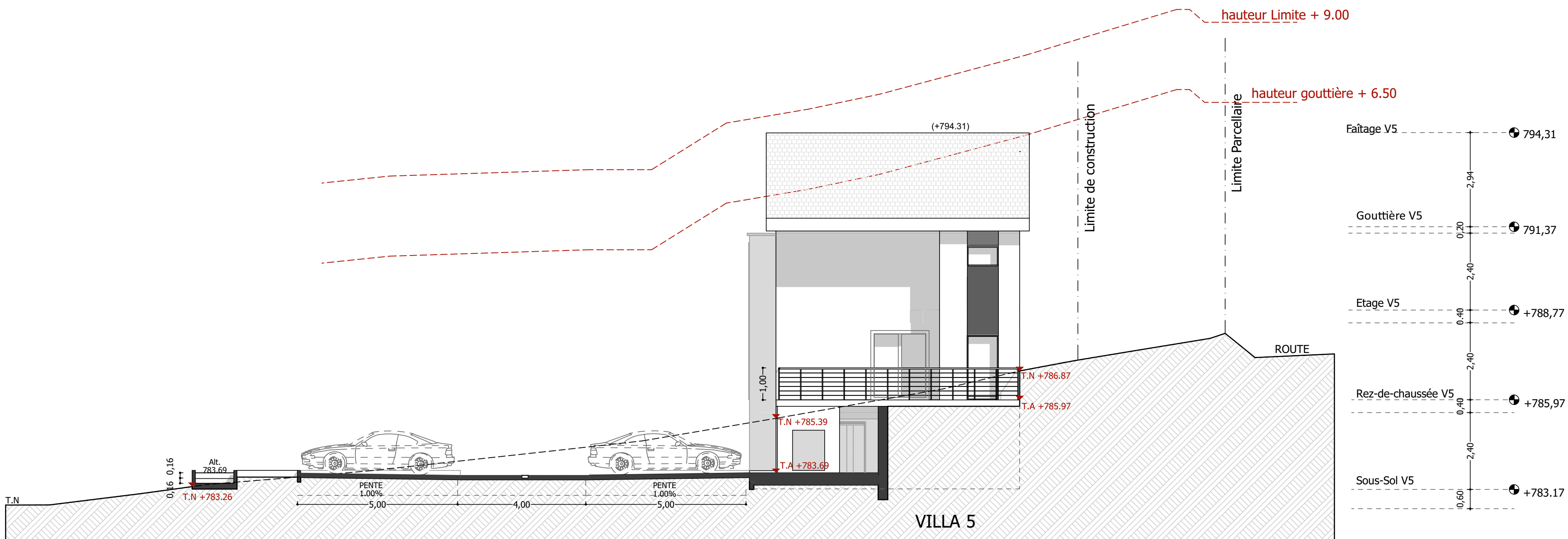
Façade Sud Villa 5 ECH: 1-100
