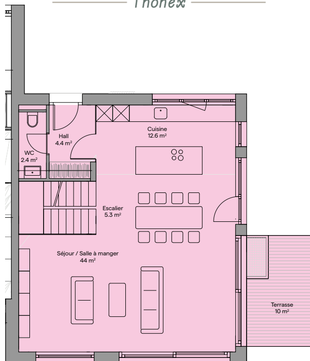
REZ-DE-CHAUSSÉE
