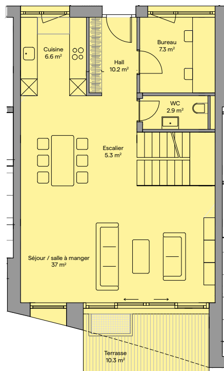
REZ-DE-CHAUSSÉE
