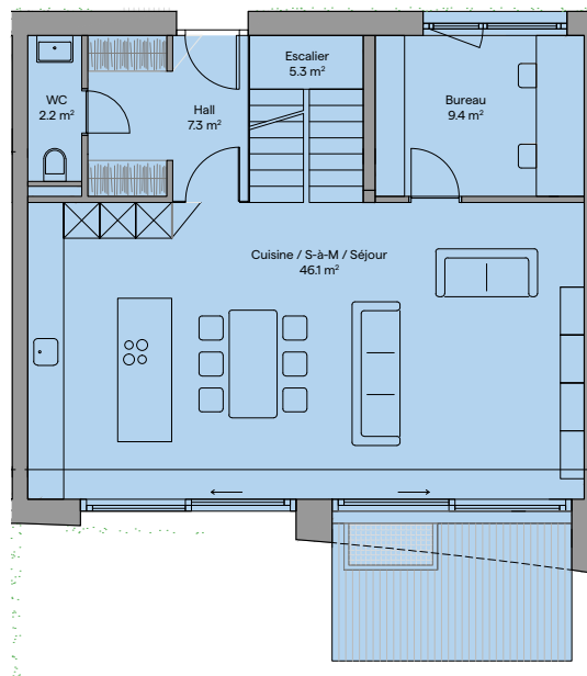
REZ-DE-CHAUSSÉE
