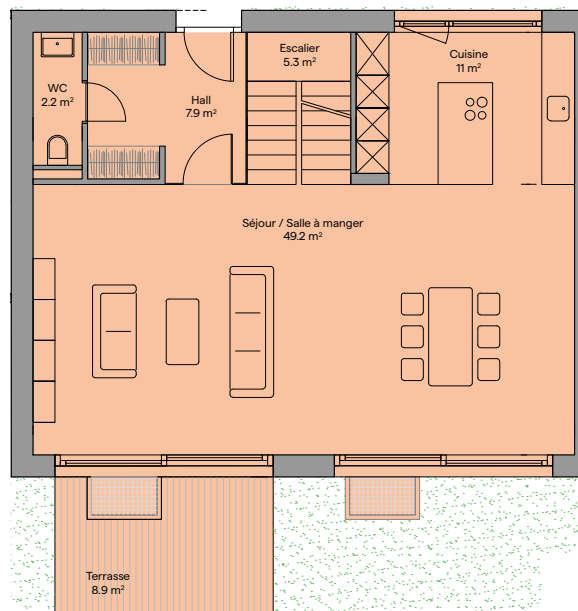
REZ-DE-CHAUSSÉE
