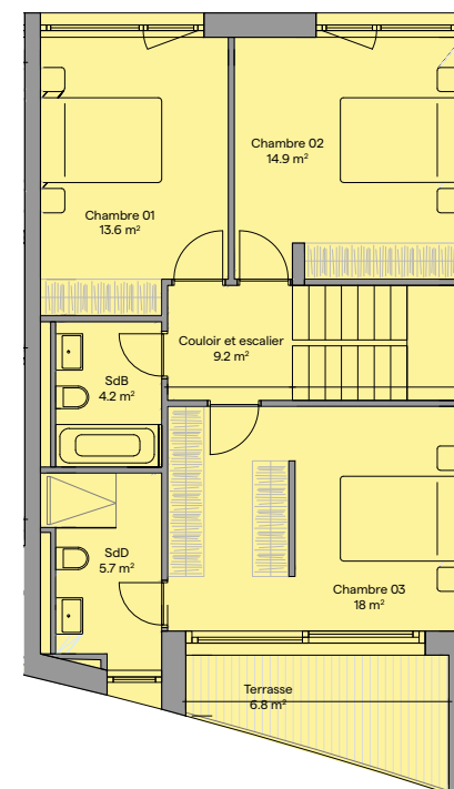
ÉTAGE
