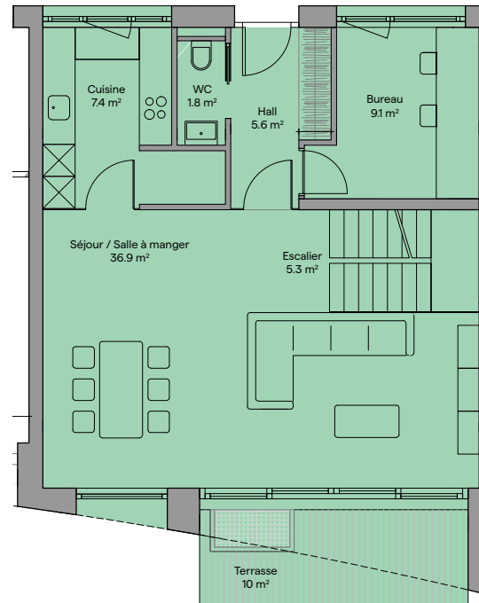
REZ-DE-CHAUSSÉE
