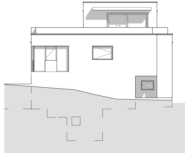
Ansicht Nord-Ost
