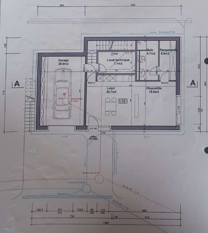
REZ-DE-CHAUSSEE INFÉRIEUR
