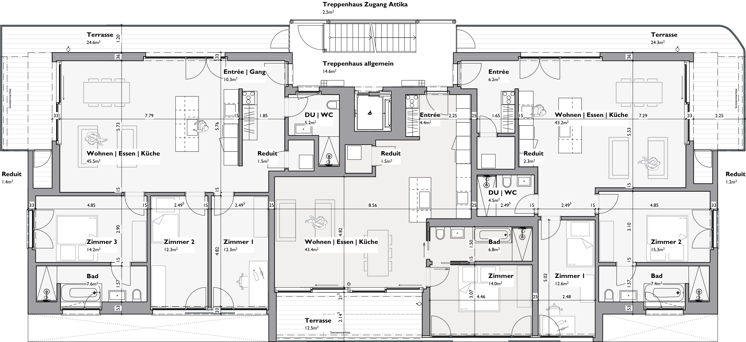
Wohnung 01.02 Obergeschoss Mitte 2.5 Zi | NF: 70.1m² gedeckte Terrasse 12.5m² Keller 12.9m²
