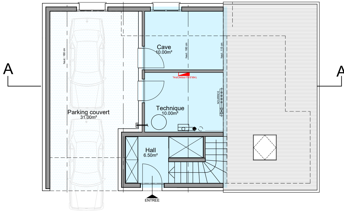
Type 2B LOT 7 - 5½ Pièces 192.00m 2 surface pondérée
