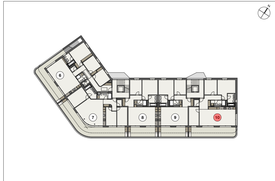
ÉTAGE 1 | 1:500
