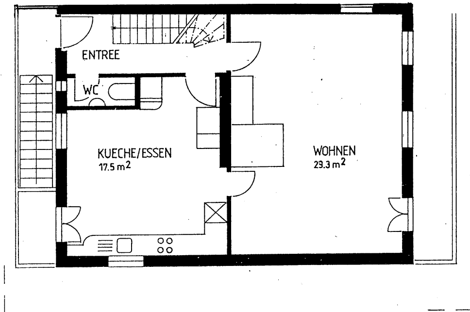
1. OBERGESCHOSS
