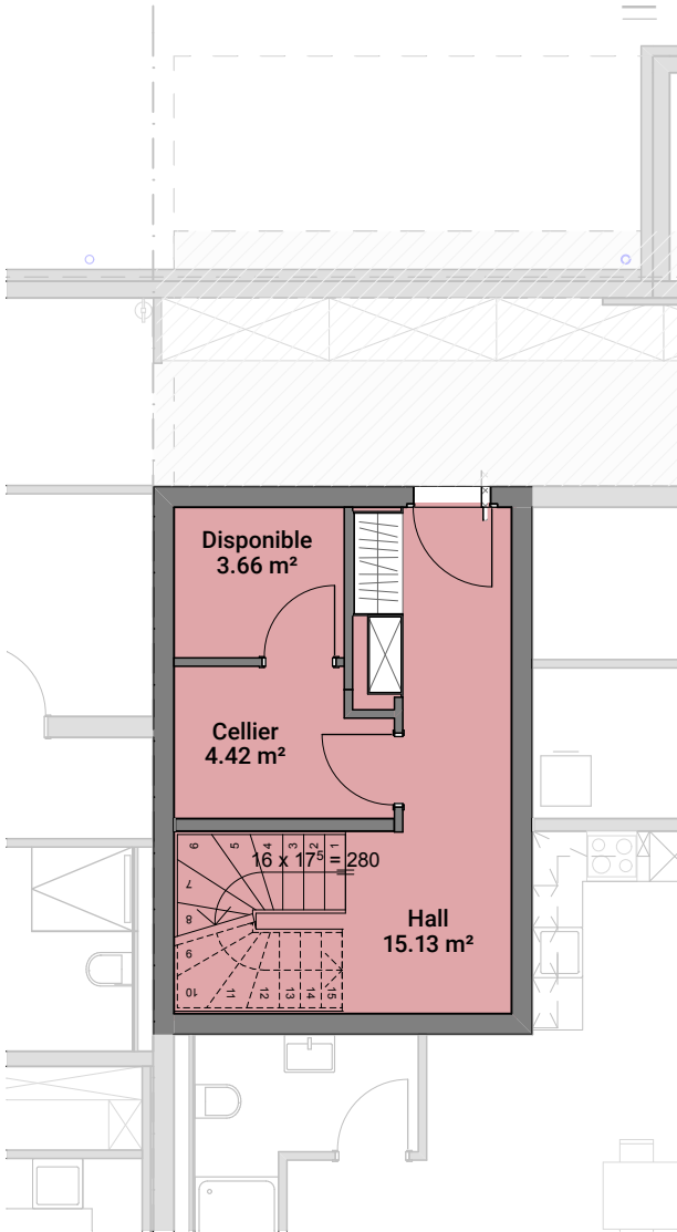
Schéma emplacement appartement
