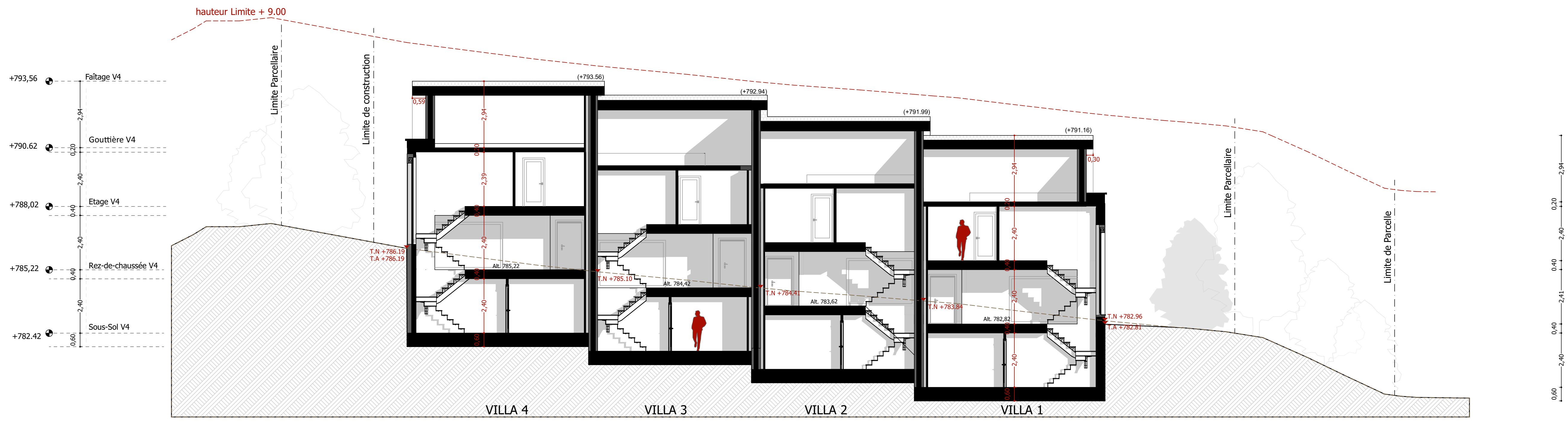
COUPE B-B' ECH: 1-100
