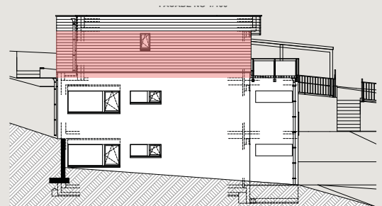
Bâtiment B1 / Façade nord-ouest
