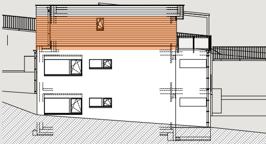
Bâtiment B2 / Façade nord-ouest
