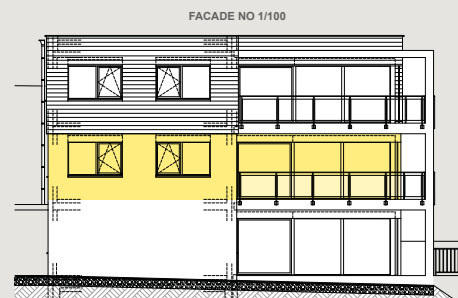
Bâtiment A1 / Façade nord-ouest
