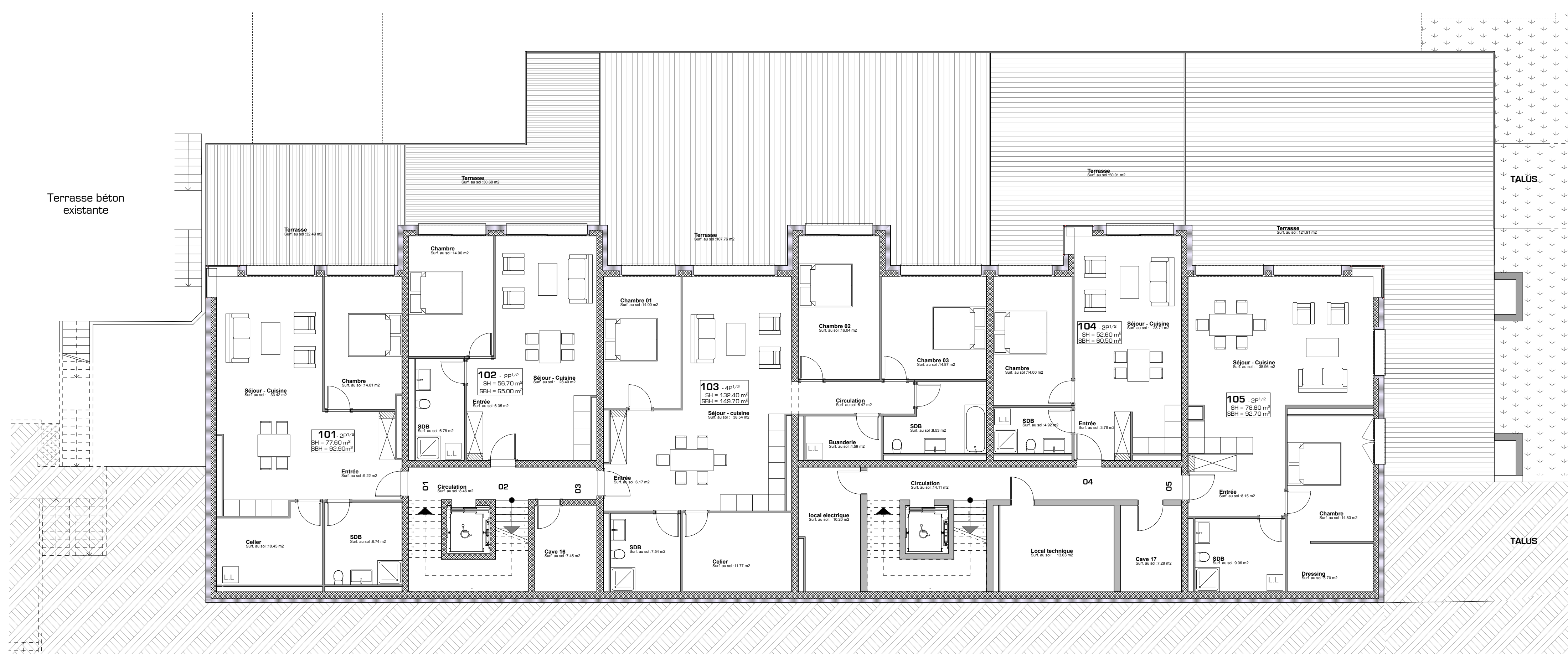
ETAGE 1 ECH. 1:100
