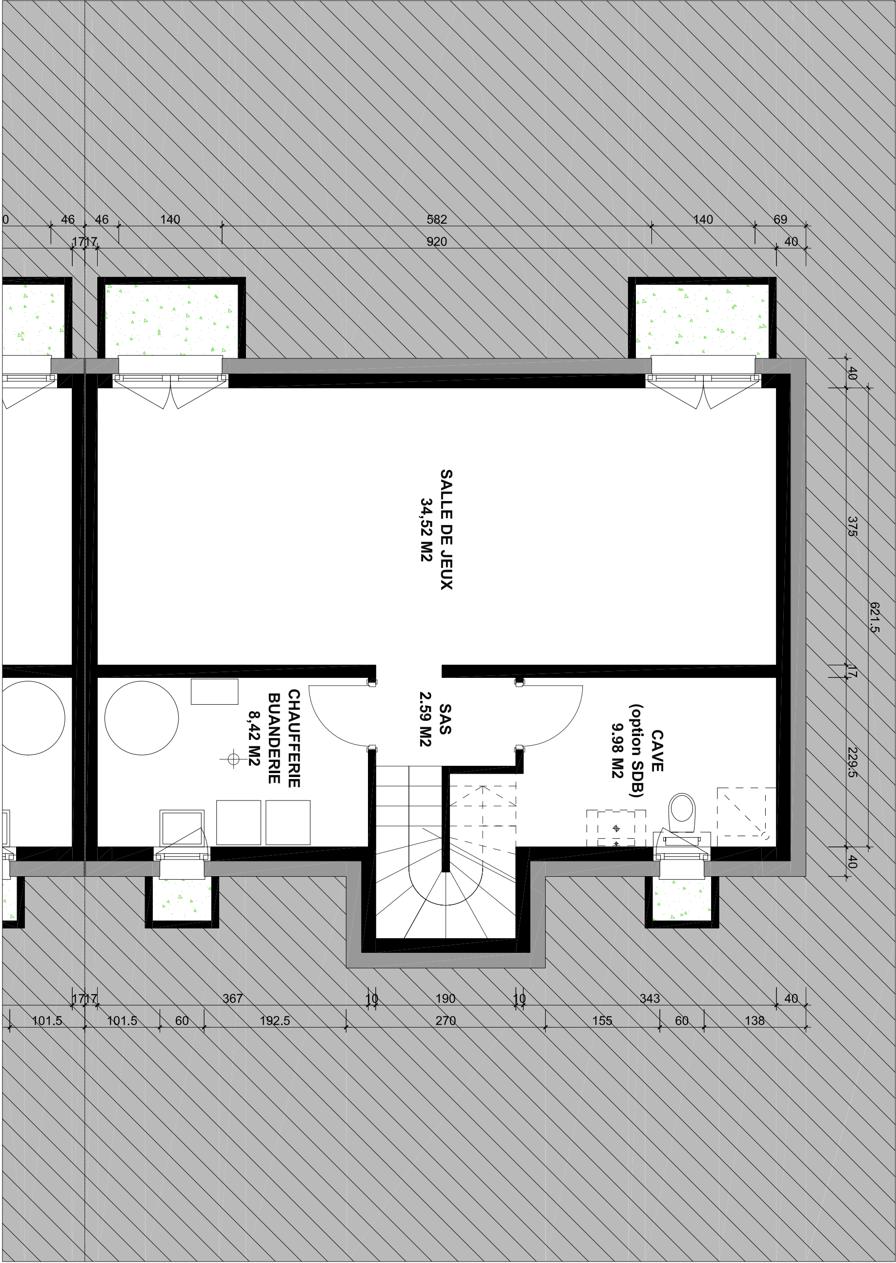
PLAN TYPE DU SOUS-SOL D'UNE VILLA - Ech. 1/50ème
