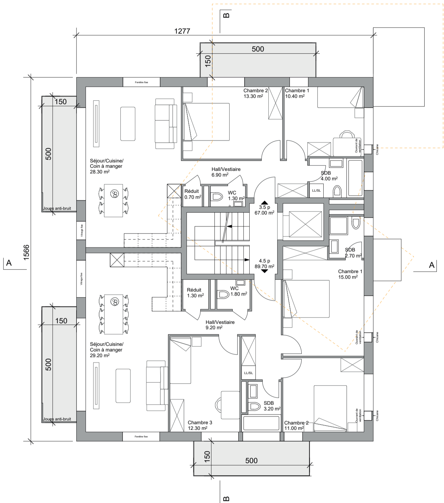
ETAGES 1 ET 2
