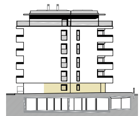
Façade nord
